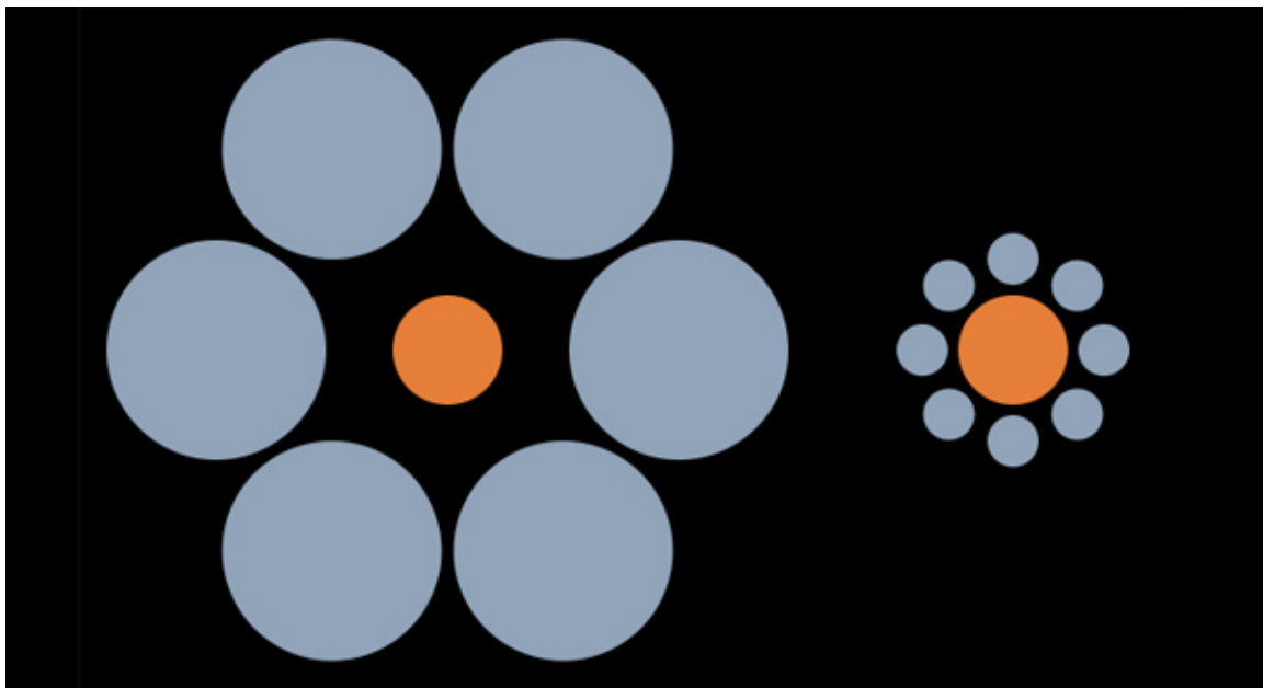
Slika2: Ebbinghaus iluzija
